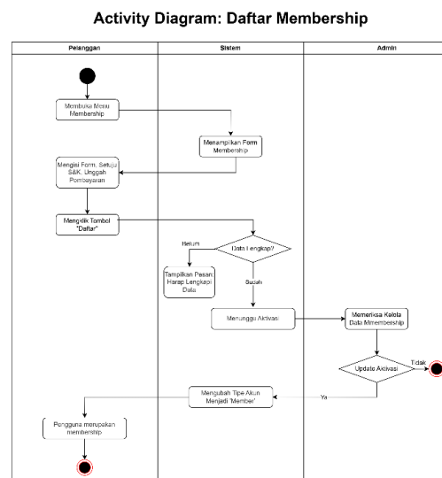
Gambar 5 Diagram Aktivitas: Daftar Membership
