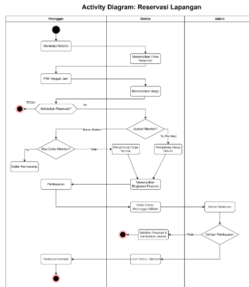
Gambar 4 Diagram Aktivitas: Reservasi Lapangan
