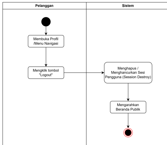
Gambar 10 Diagram Aktivitas: Logout
