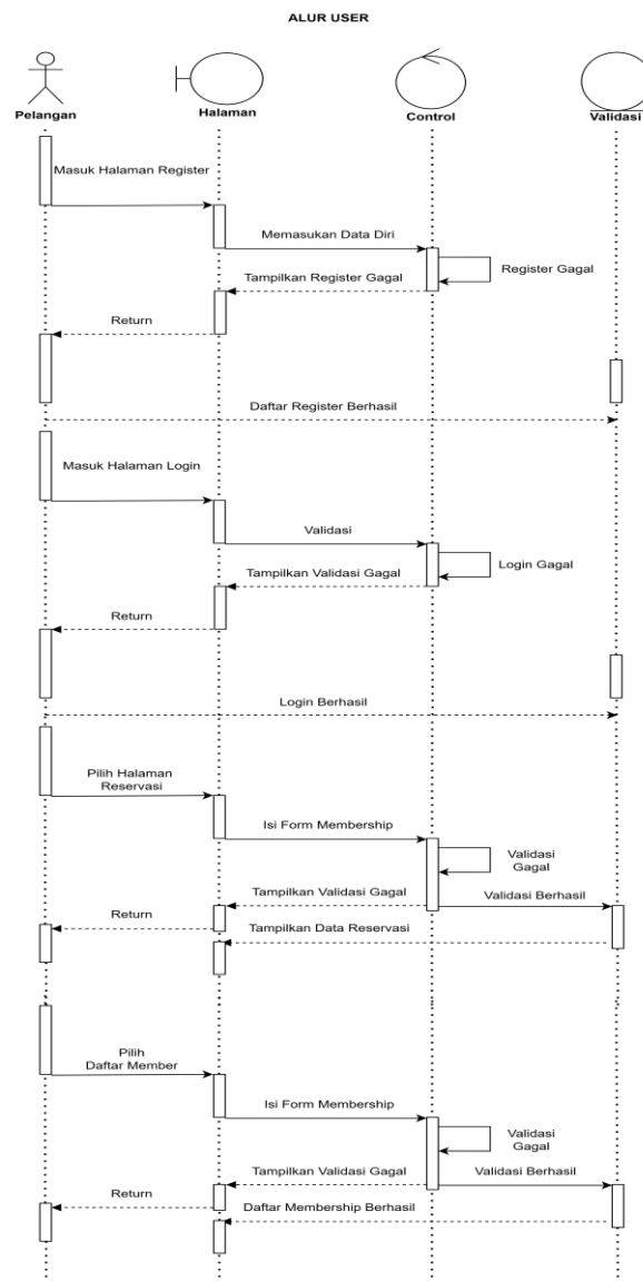
Gambar 11 Diagram Sekuens Pelanggan
