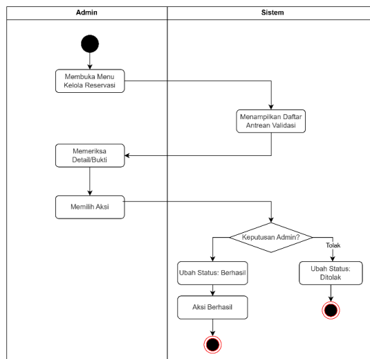
Gambar 7 Diagram Aktivitas: Kelola Reservasi
